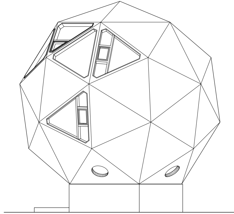
東立面图
