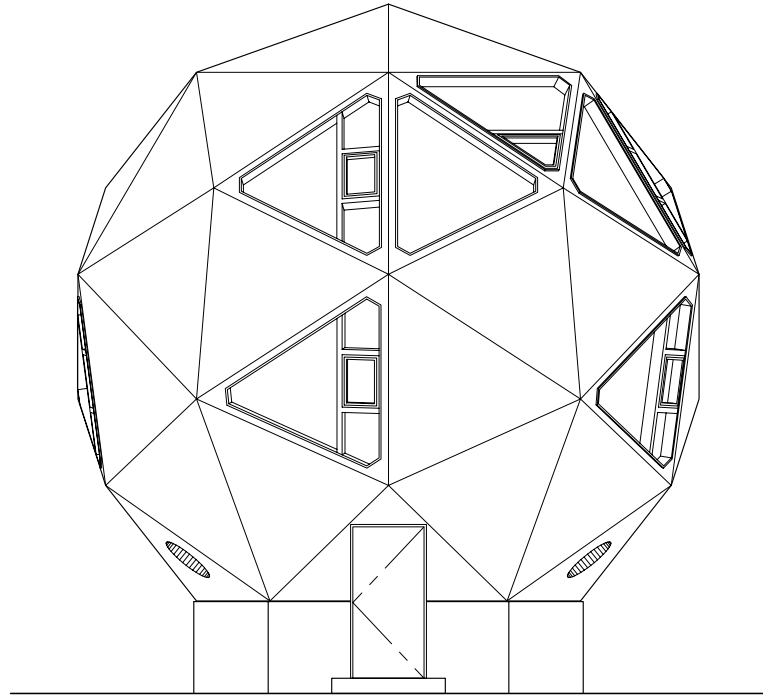
南立面图
