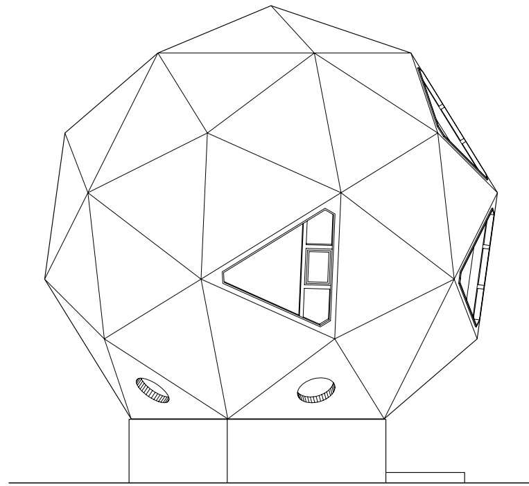
西立面图
