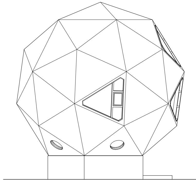
西立面图
